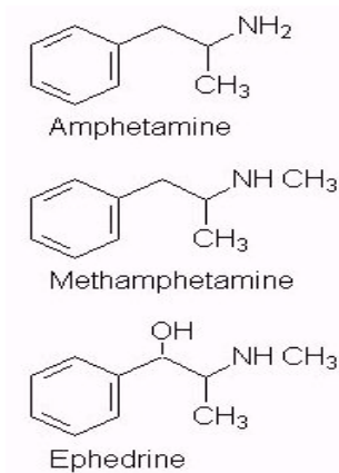
Gambar 4.2. Struktur kimia Amfetamin, Metamphetamin, dan precursornya Ephedrin
